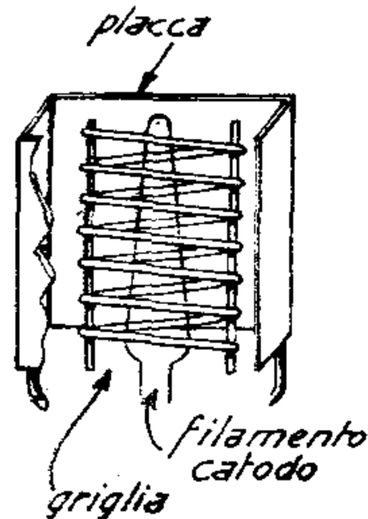
Triodo a riscaldamento diretto
