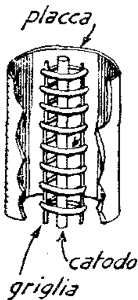
Triodo a riscaldamento indiretto
